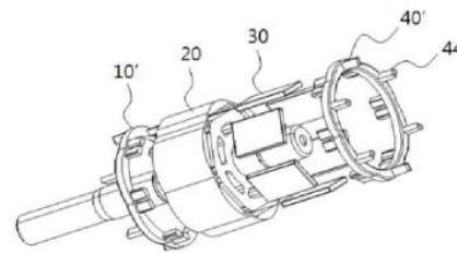
<마그넷 고정 구조체를 포함하는 모터>
